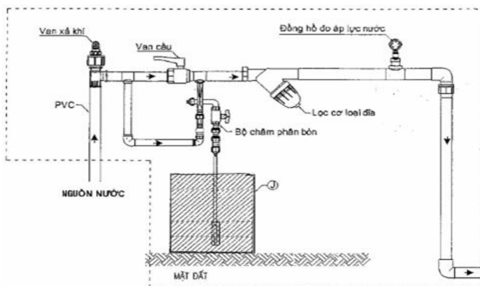
Hình 3.3: Sơ đồ lắp đặt bộ điều khiển trung tâm
