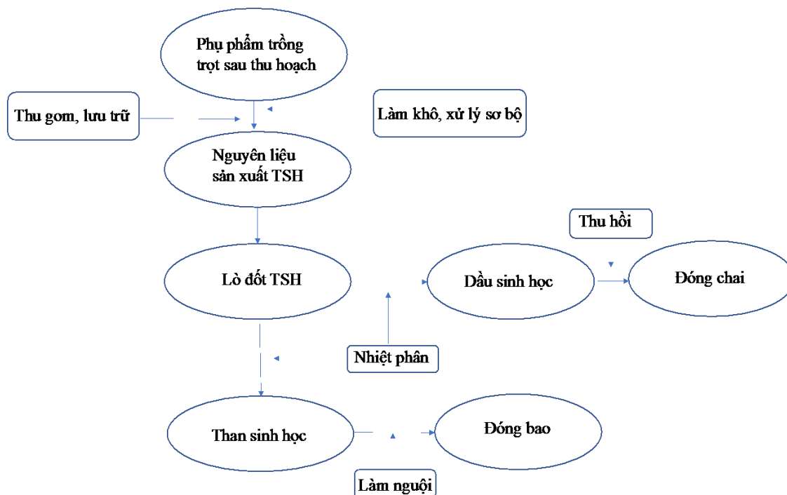
Hình 2.17. Sơ đồ quy trình sản xuất than sinh học bằng lò đốt cải tiến
