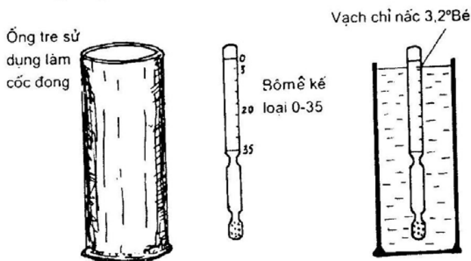
Hình 4: Cốc đựng, Bômê kế và cách sử dụng
